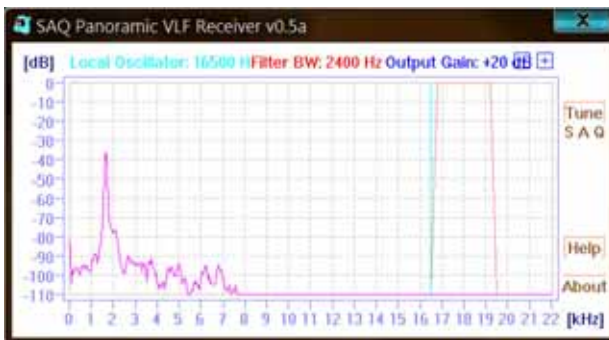
Screenshot van software VLF ontvanger
